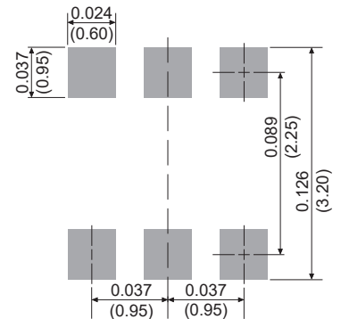
SOT-23 6L-1/SOT-26-1
