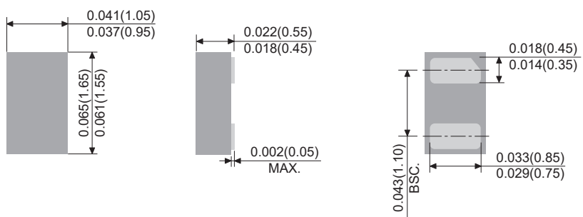
DFN1610-2L
