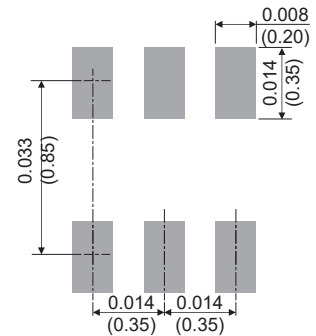
DFN1010B-6L
