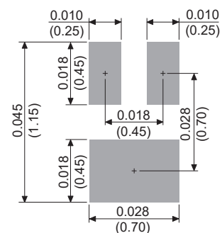
DFN1610-2L
