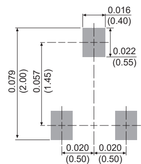
SOT-523
