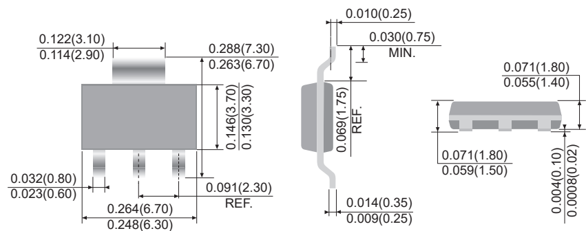
SOT-223
