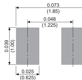
DFN1610-2L
