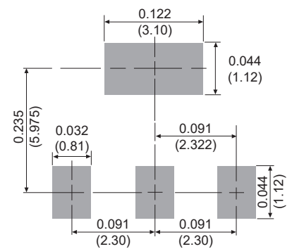
SOT-89
