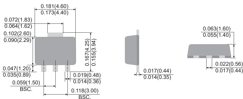
SOT-89
